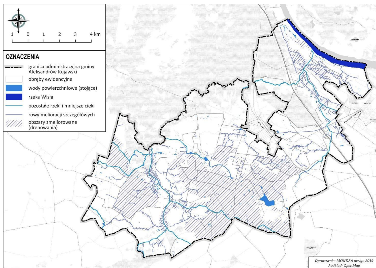
Ryc. 1. Szczegółowe urządzenia melioracji wodnych
